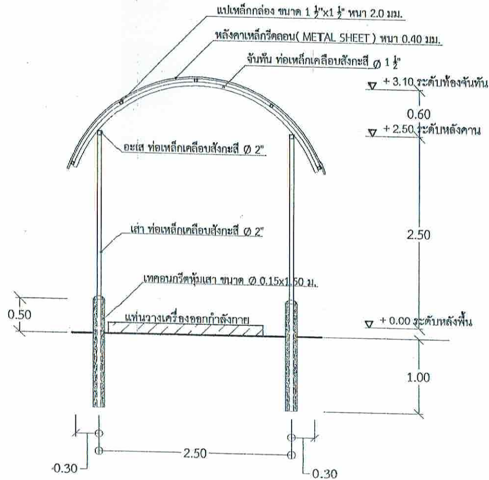
รูปตัด A - A (หลังคาคลุมเครื่องออกกำลังกาย)
