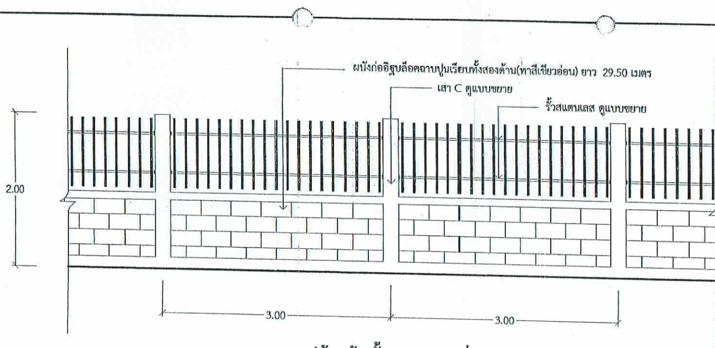
รูปด้านข้างรั้ว คสล.(ช่วงที่ 1)
