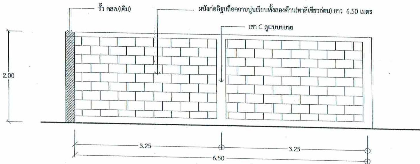
รูปด้านข้างรั้ว คสล.(ช่วงที่ 2)
