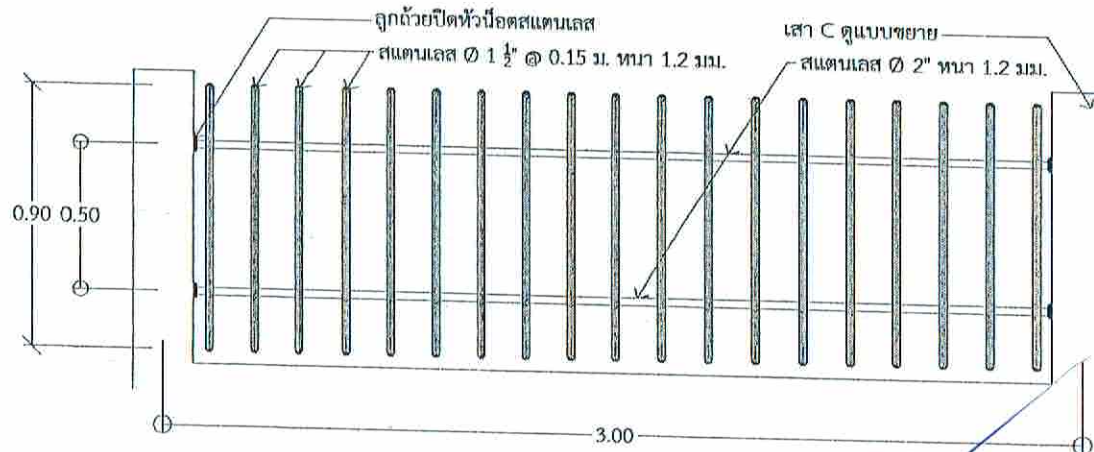
ขยายรั้วสแตนเลส
