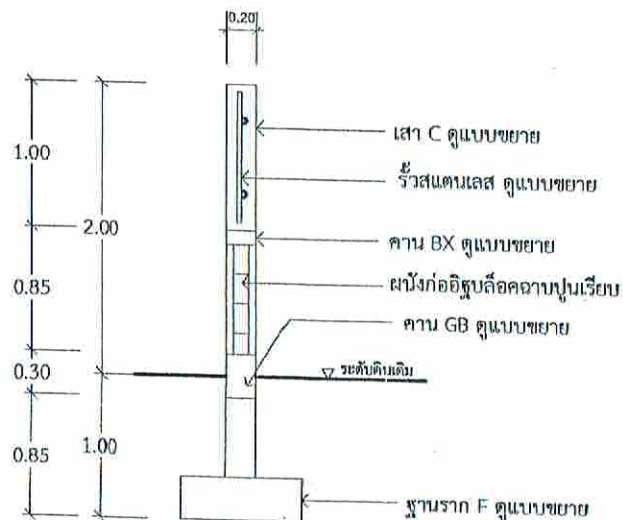
รูปตัดรั้ว คสล.(ช่วงที่ 1)
