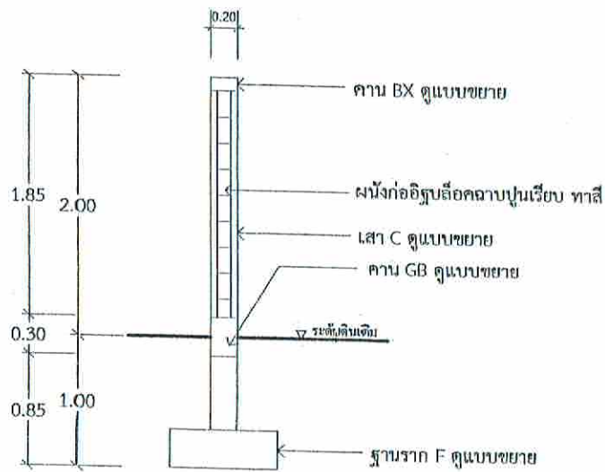
รูปตัดรั้ว คสล.(ช่วงที่ 2)
